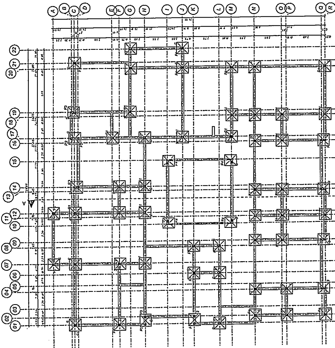
PLAN DES FONDATIONS
